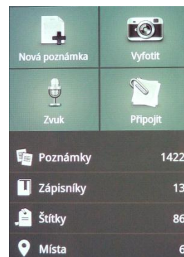
Obrázek 2 - Android klient
