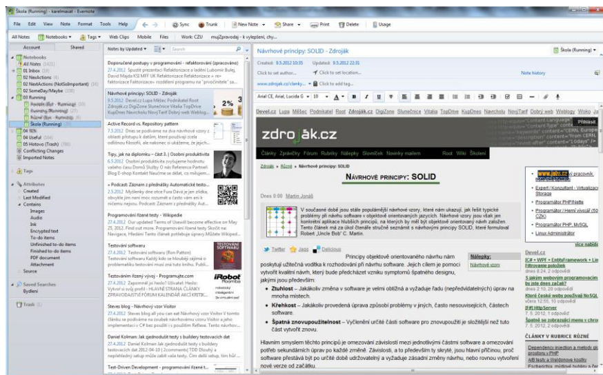
Obrázek 1 - Windows klient
